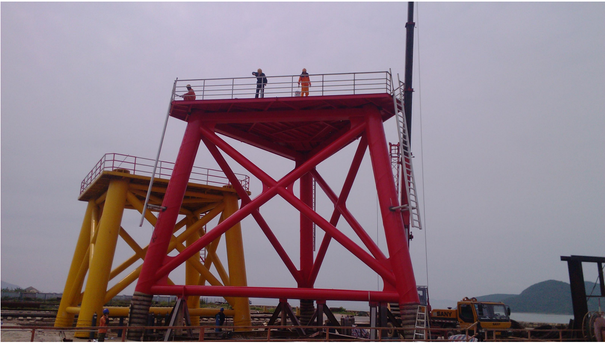
风电的导管架
